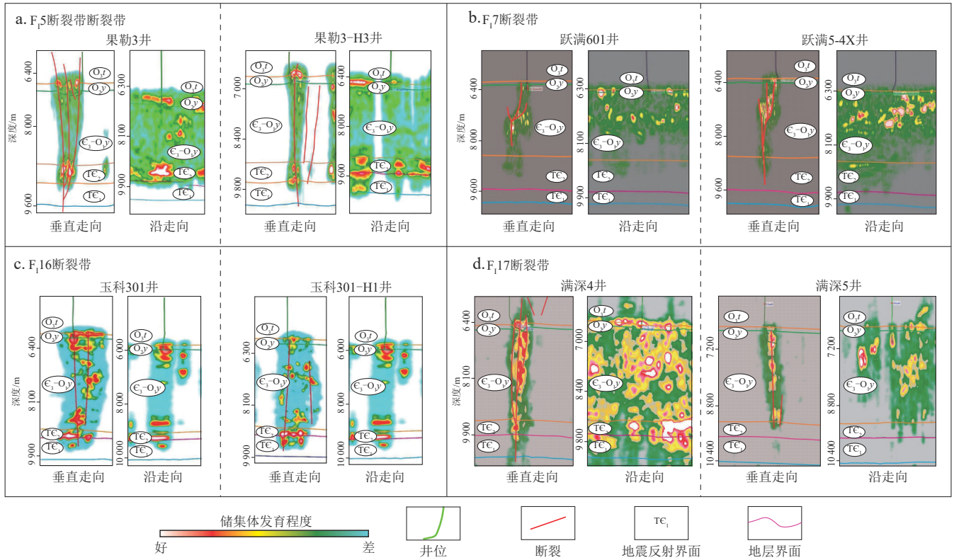
图9 富满地区典型走滑断裂带储层空间分布特征
